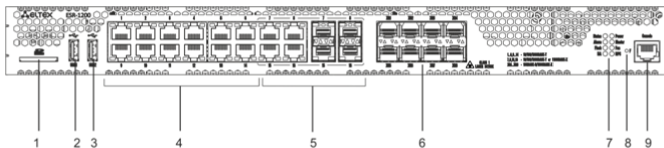
Рисунок 18 – Передняя панель ESR-1200
