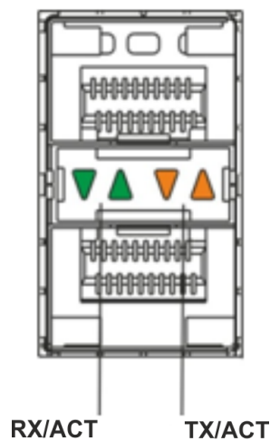
Рисунок 53 – Расположение индикаторов оптических интерфейсов
