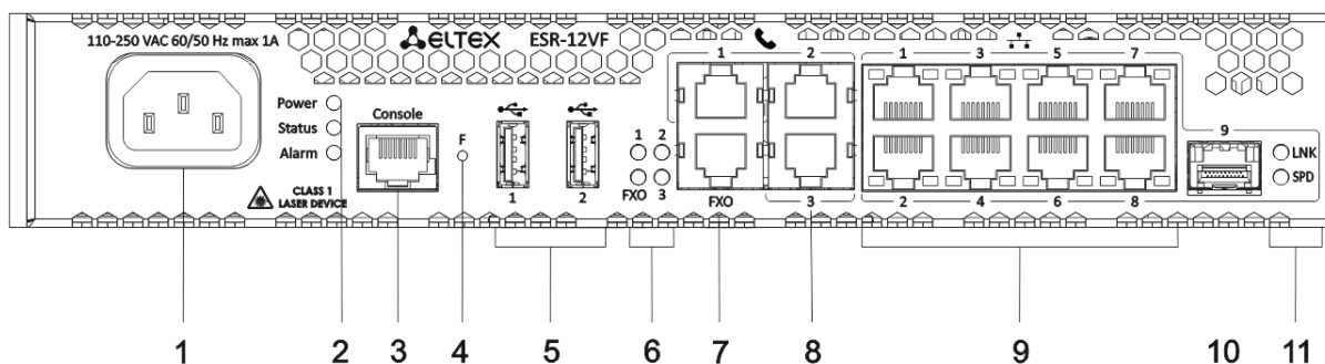
Рисунок 43 – Передняя панель ESR-14VF, ESR-12VF
