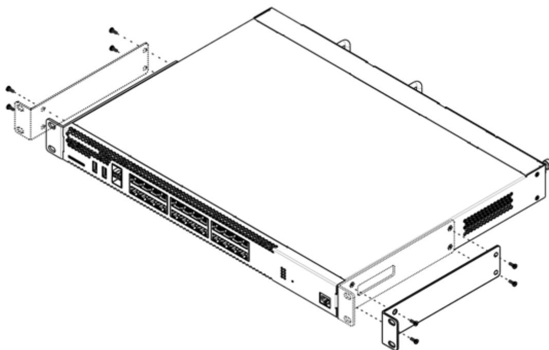
Рисунок 67 – Крепление кронштейнов
