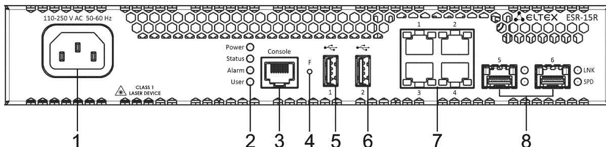
Рисунок 39 – Передняя панель ESR-15R
