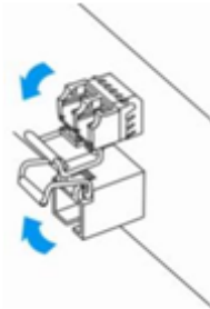
Рисунок 75 – Открытие защелки SFP-трансиверов
