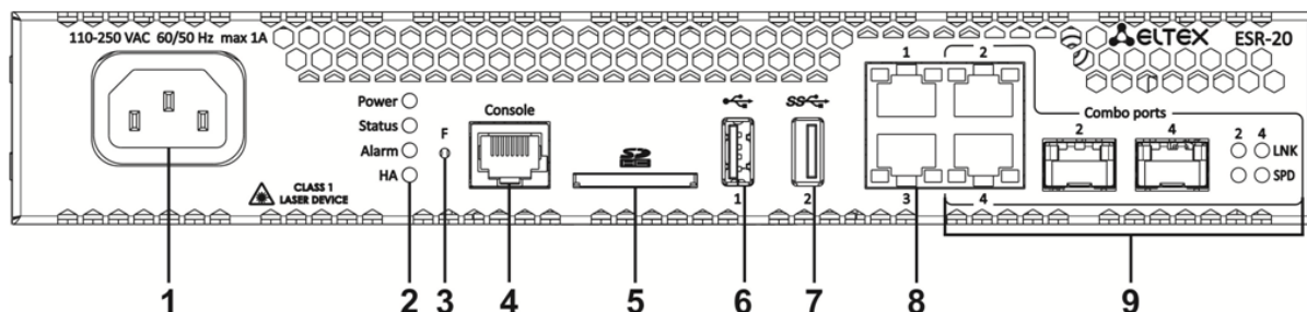
Рисунок 41 – Передняя панель ESR-20
