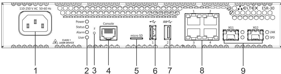
Рисунок 40 – Передняя панель ESR-30
