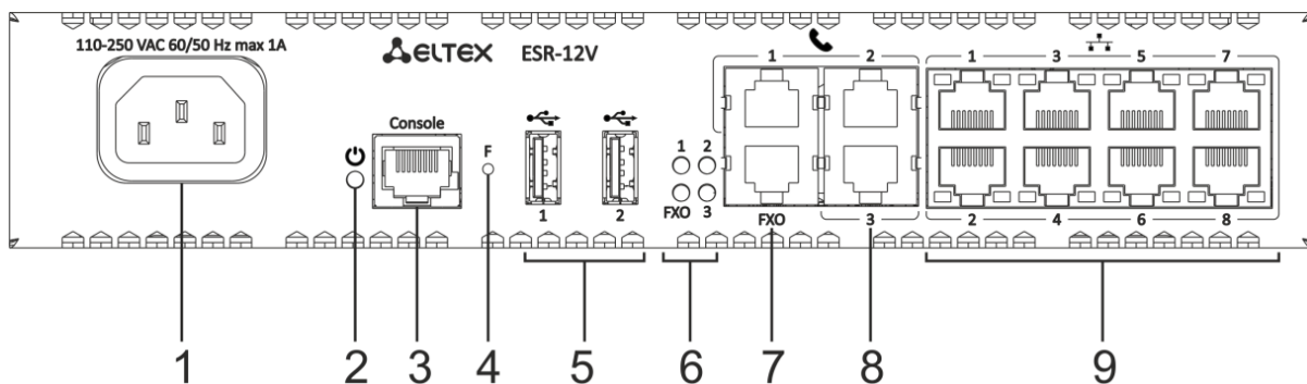
Рисунок 51 – Передняя панель ESR-12V
