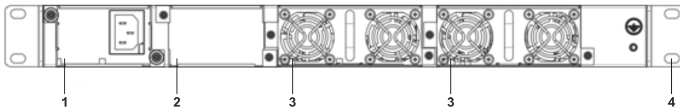
Рисунок 28 – Задняя панель ESR-1000
