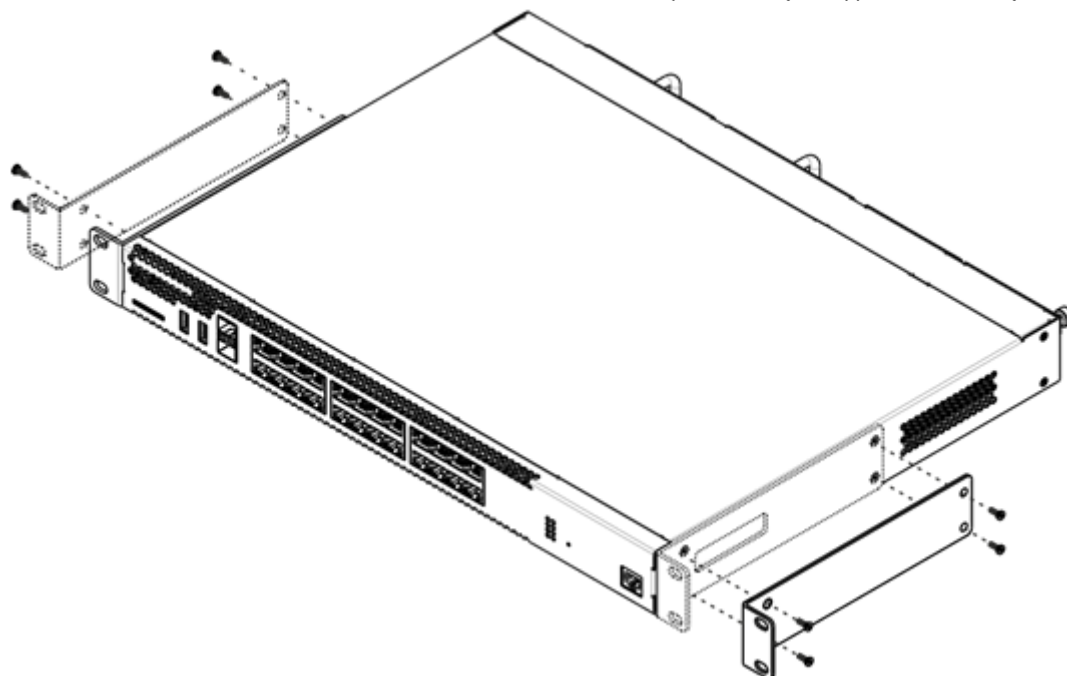
Рисунок 69 – Крепление кронштейнов
