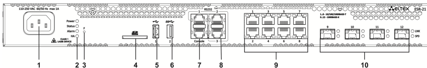
Рисунок 36 – Передняя панель ESR-21
