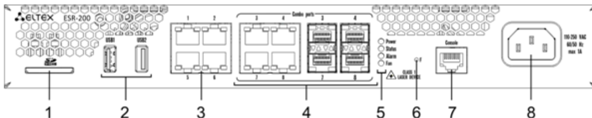
Рисунок 31 – Передняя панель ESR-200
