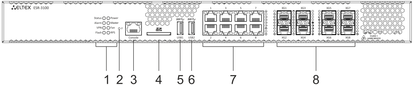
Рисунок 13 – Передняя панель ESR-3100
