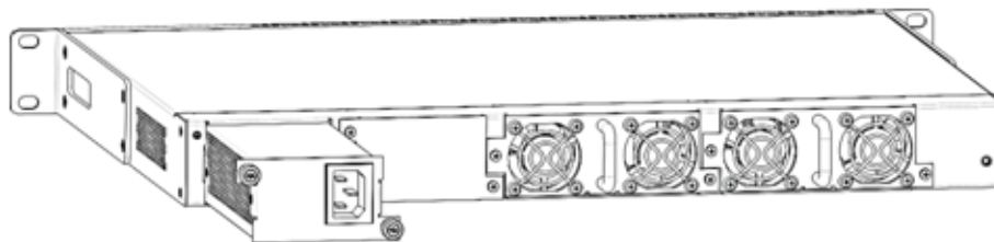
Рисунок 71 – Установка модулей питания
