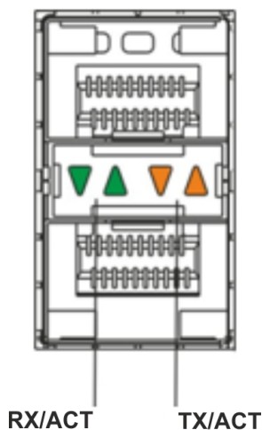
Рисунок 61 – Расположение индикаторов оптических интерфейсов
