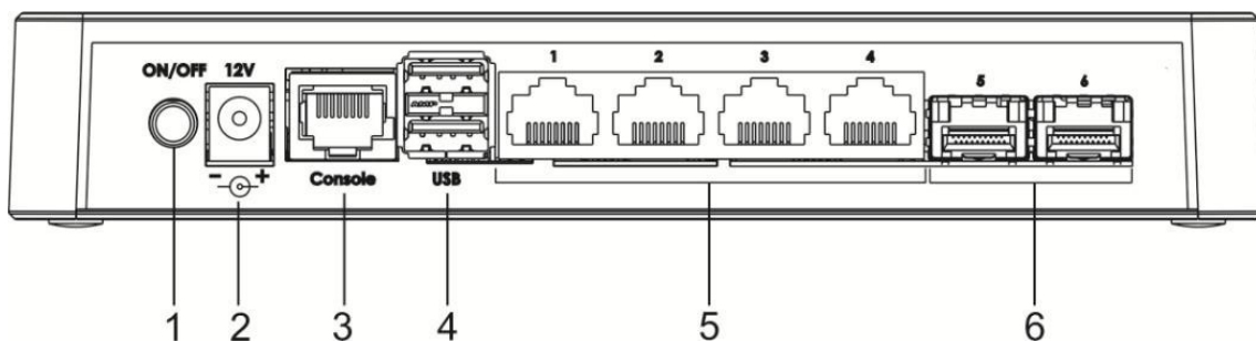
Рисунок 55 – Задняя панель ESR-10
