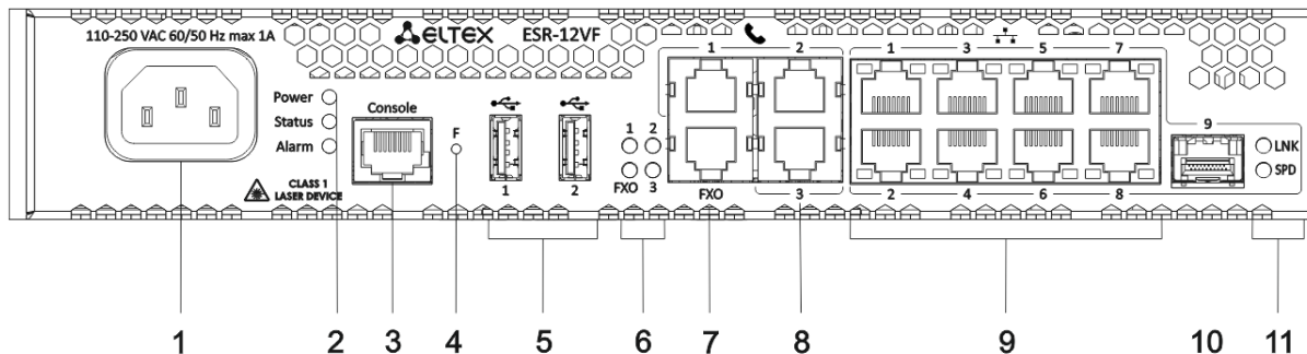
Рисунок 47 – Передняя панель ESR-14VF, ESR-12VF
