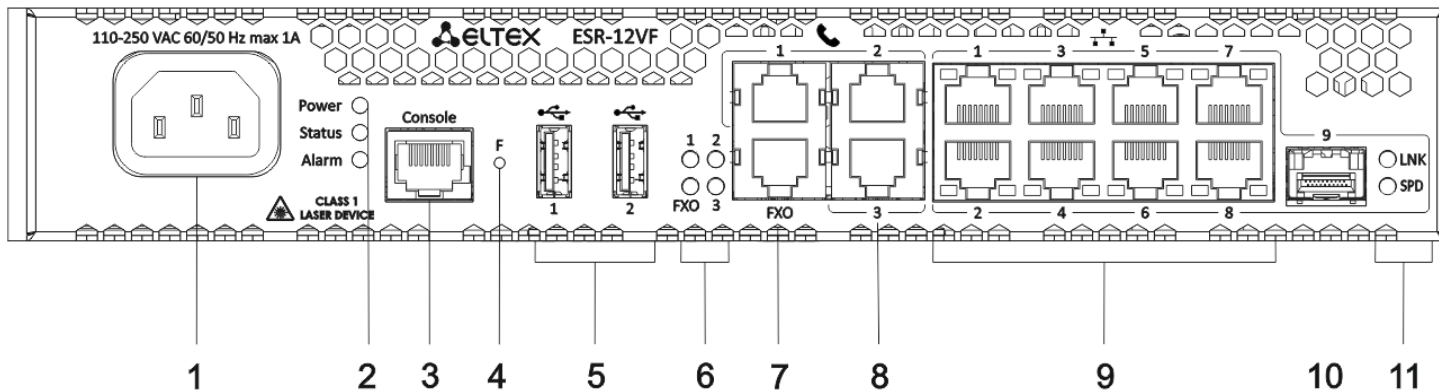
Рисунок 27 – Передняя панель ESR-12VF, ESR-14VF
