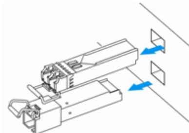
Рисунок 52 – Извлечение SFP-трансиверов
