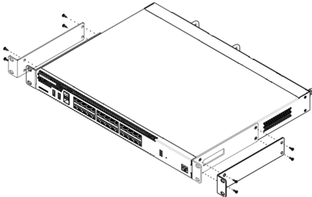
Рисунок 45 – Крепление кронштейнов
