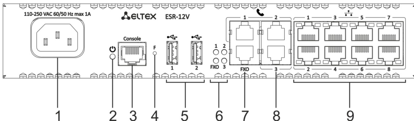
Рисунок 31 – Передняя панель ESR-12V
