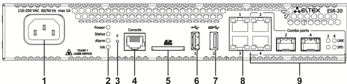
Рисунок 23 – Передняя панель ESR-20
