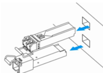
Рисунок 52 – Извлечение SFP-трансиверов
