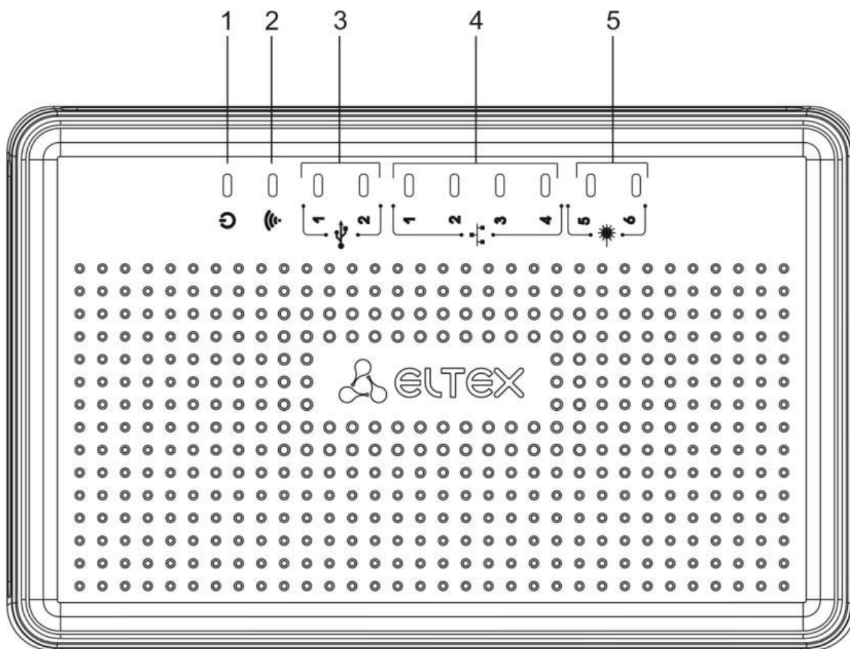
Рисунок 37 – Верхняя панель маршрутизатора ESR-10
