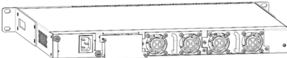
Рисунок 48 – Установка заглушки
