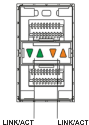
Рисунок 40 – Расположение индикаторов оптических интерфейсов
