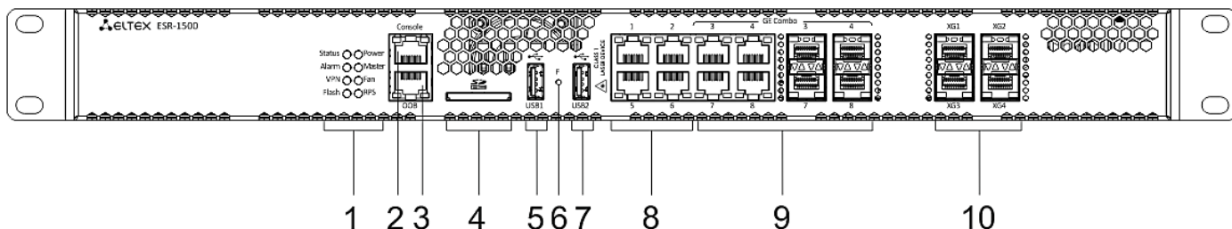
Рисунок 5 – Передняя панель ESR-1500
