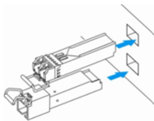
Рисунок 49 – Установка SFP-трансиверов
