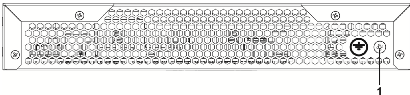
Рисунок 24 – Задняя панель ESR-20
