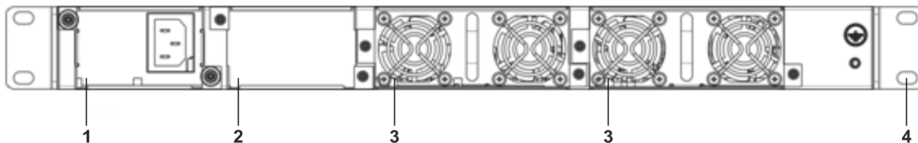
Рисунок 11 – Задняя панель ESR-1200, ESR-1000
