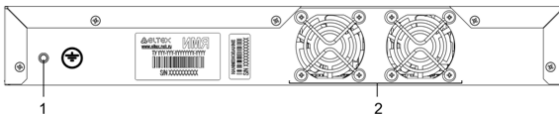
Рисунок 16 – Задняя панель ESR-200, ESR-100
