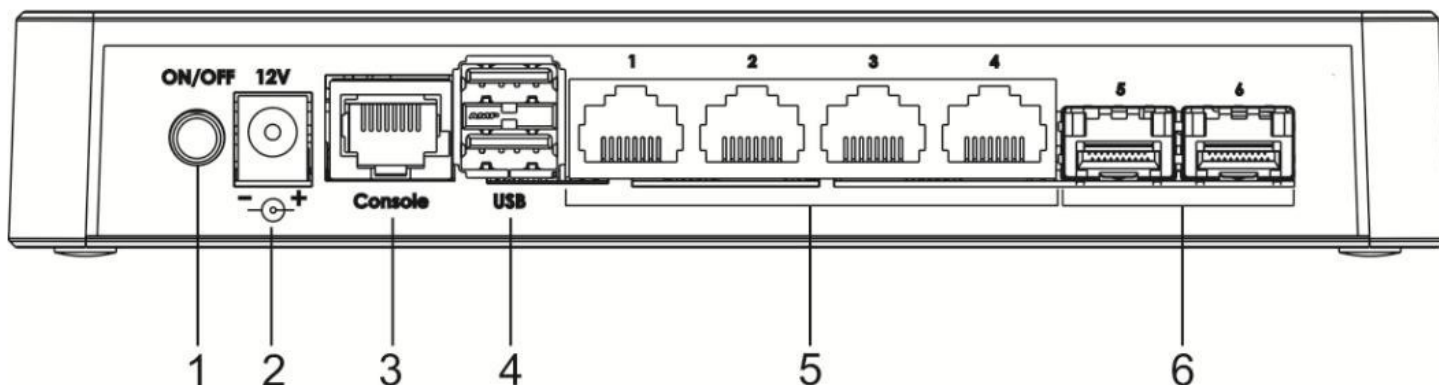
Рисунок 35 – Задняя панель ESR-10
