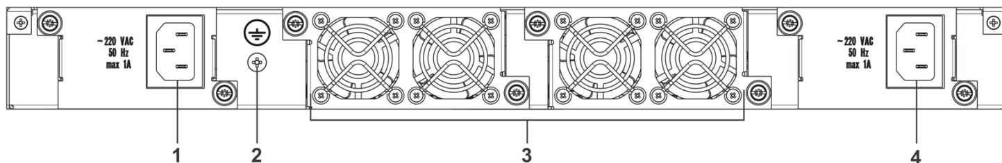
Рисунок 6 – Задняя панель ESR-1500
