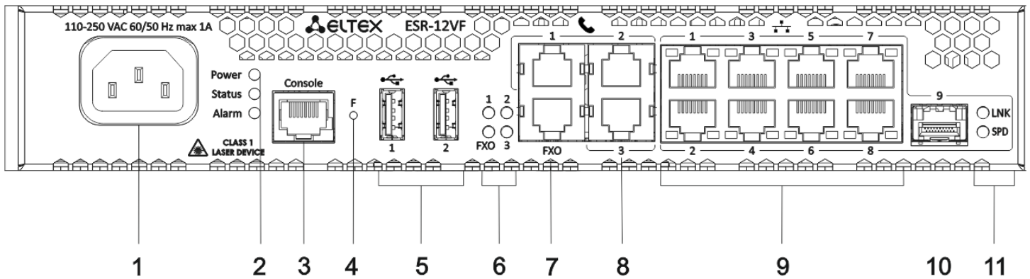
Рисунок 27 – Передняя панель ESR-12VF
