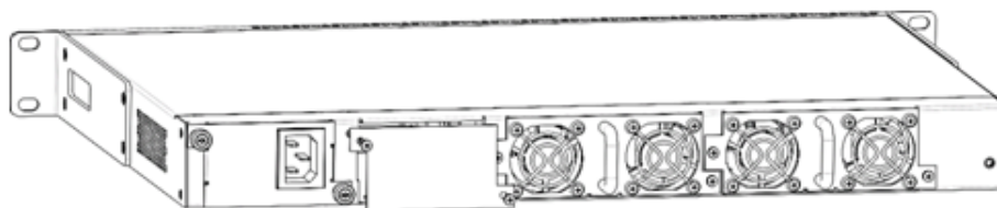
Рисунок 93 – Установка заглушки
