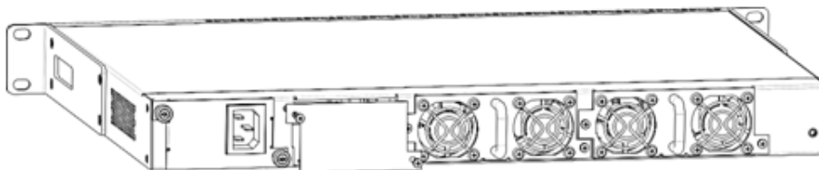
Рисунок 93 – Установка заглушки
