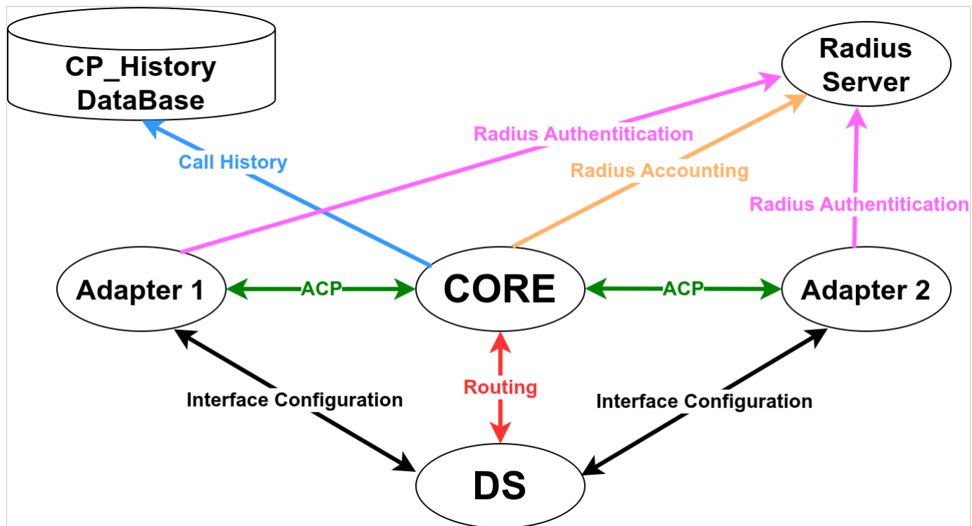
Рисунок 3 – Обмен сообщениями в системе ECSS-10 в рамках обслуживания вызова
