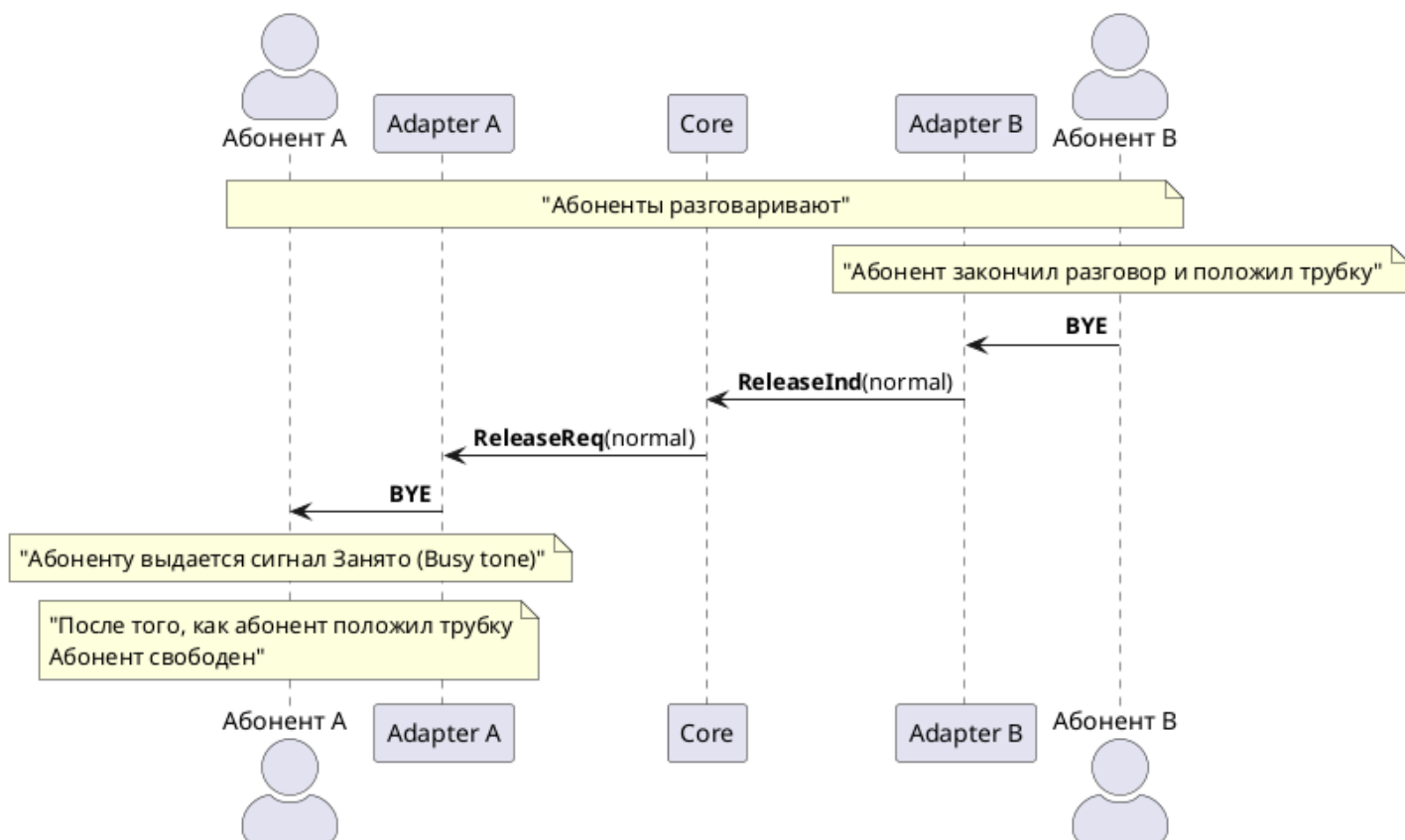
Рисунок 15 — Разъединение вызова по инициативе абонента Б, упрощенный вид
