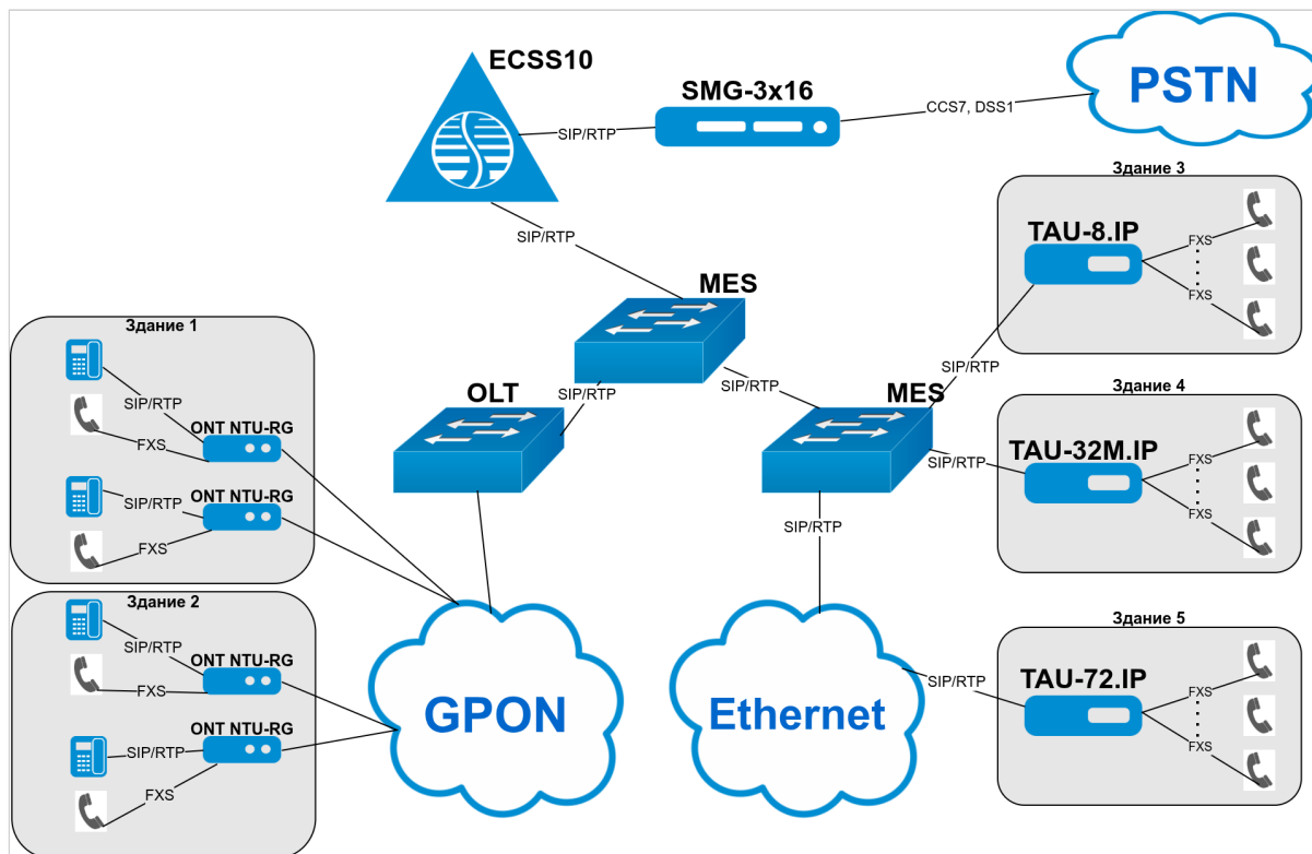
Рисунок 3 — Пример построения городского узла связи на основе ECSS-10
