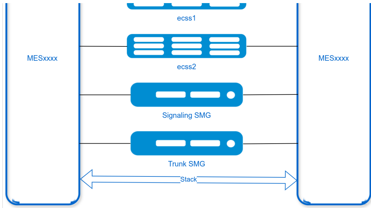
Рисунок 2 — Схема включения оборудования ECSS-10:
