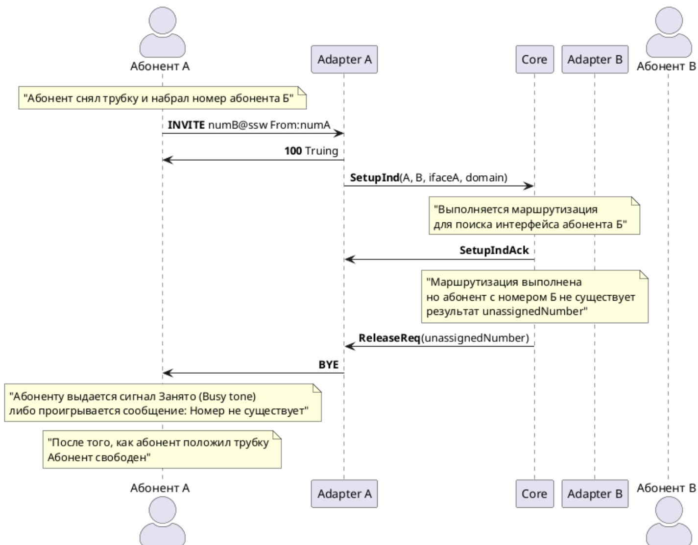
Рисунок 16 — Неуспешный вызов по причине того, что номер Б не существует
