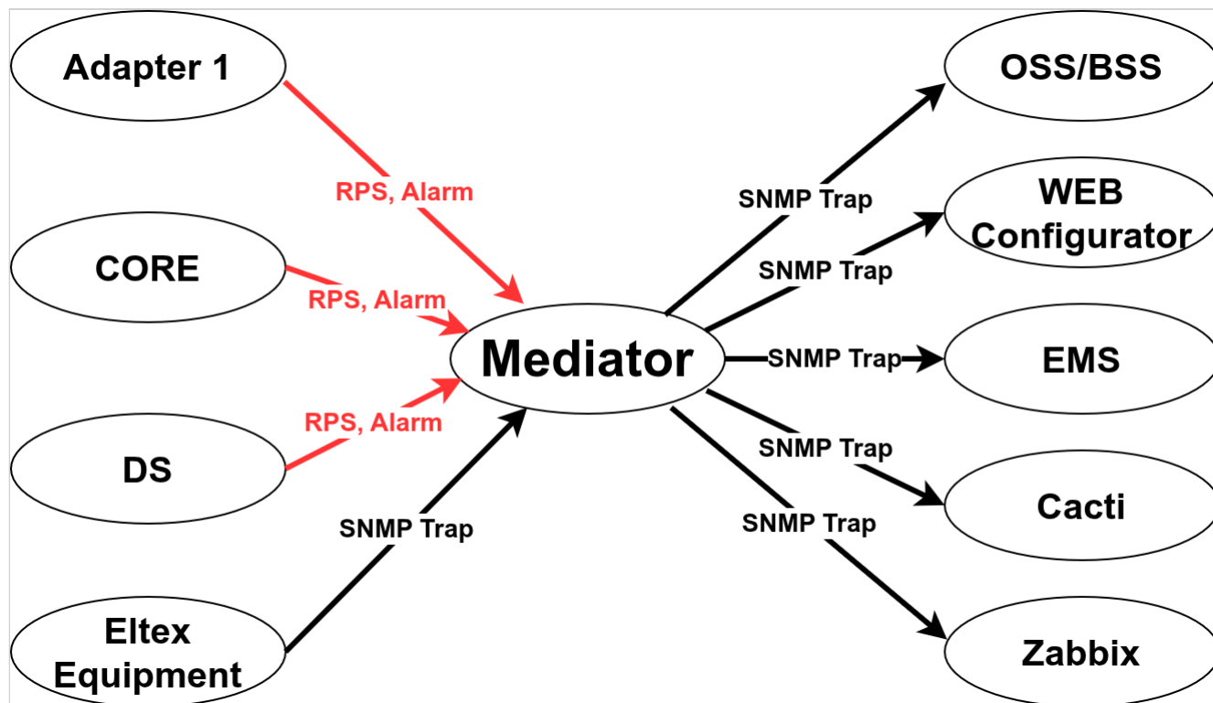
Рисунок 4 – Пути отправки сообщения об аварии системе ECSS-10
