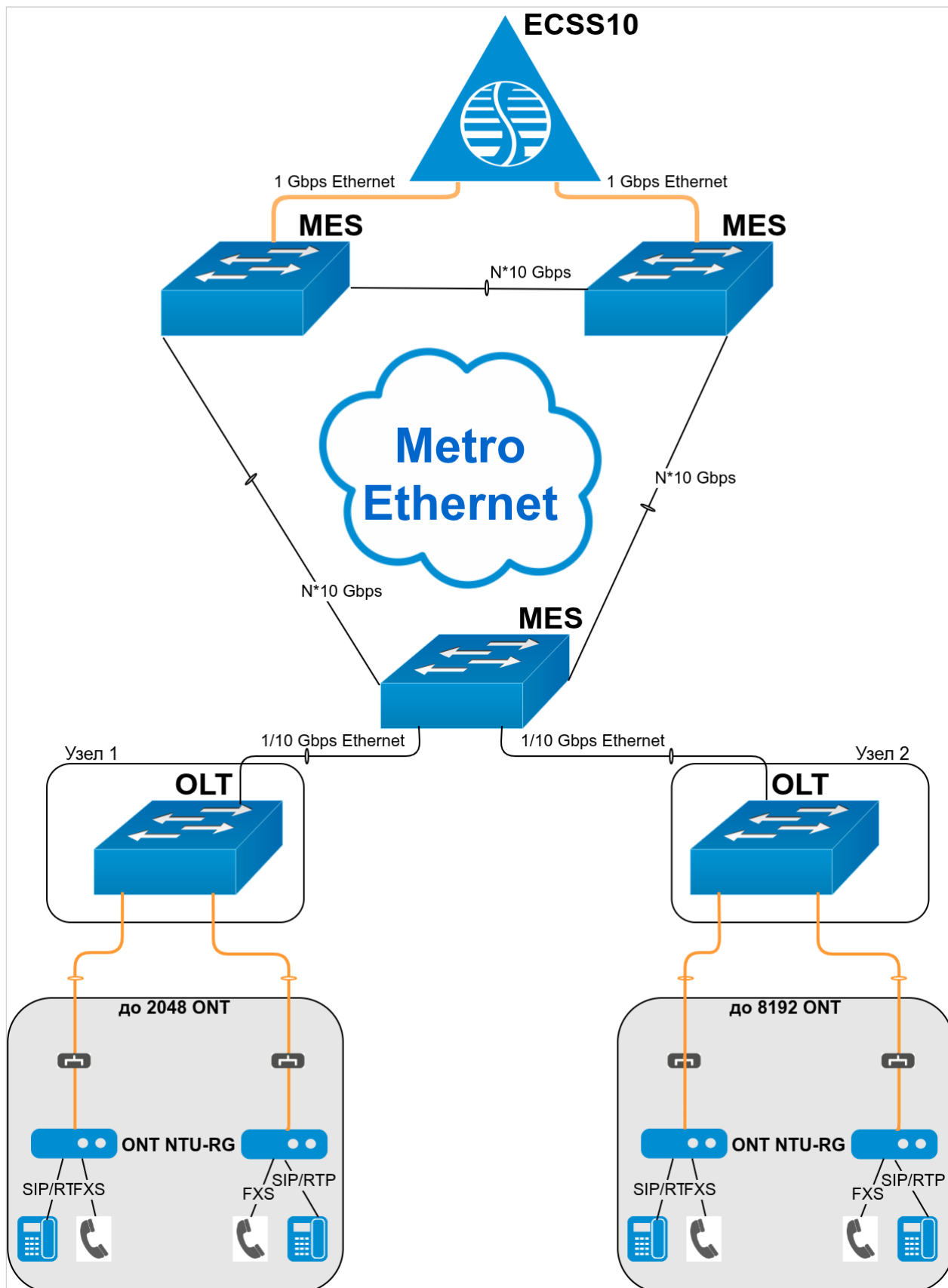
Рисунок 4 — Пример построения современной IP-сети с использованием на "последней миле" технологии PON
