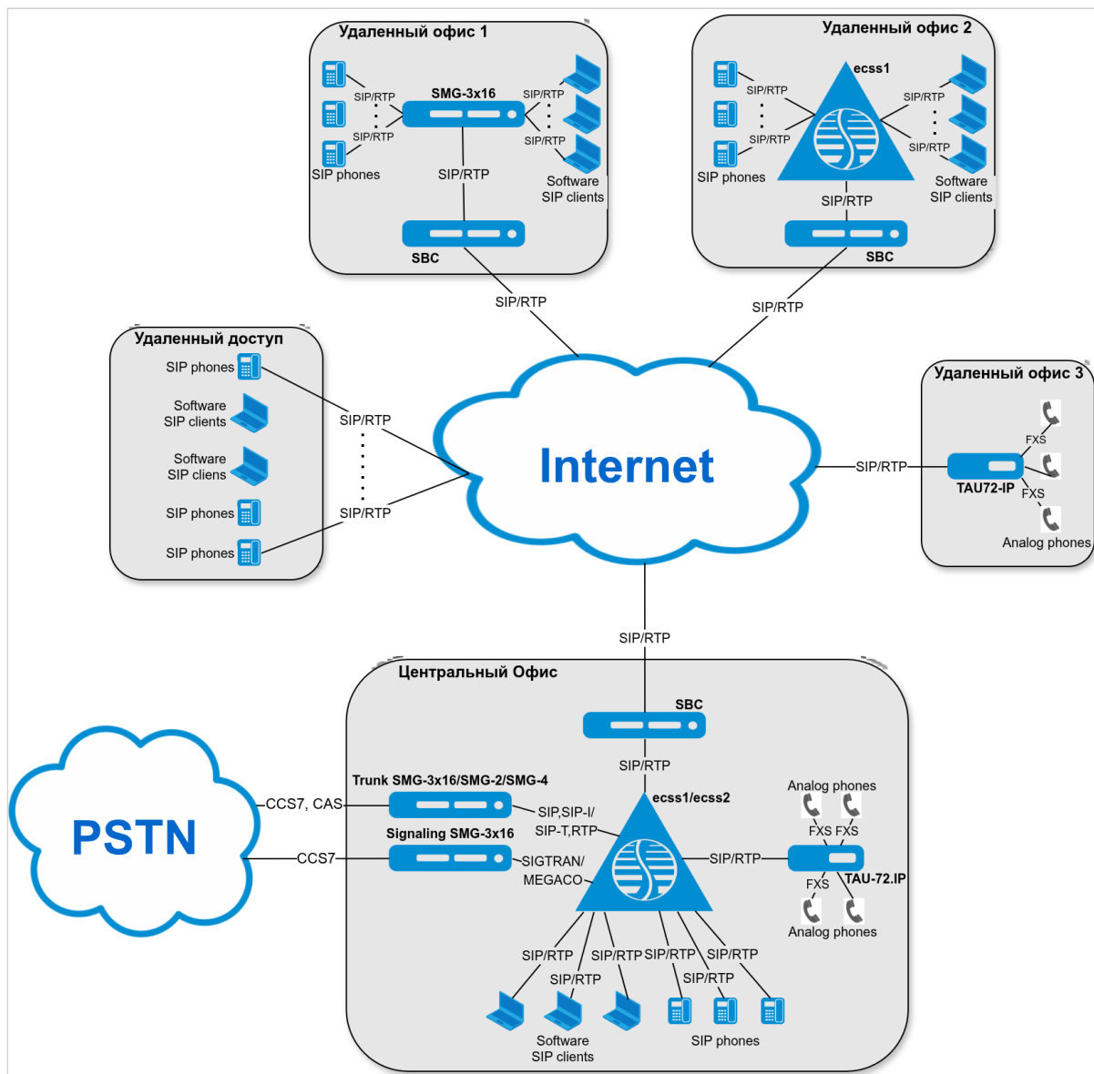
Рисунок 1 — Пример построения распределённой корпоративной сети на основе ECSS-10
