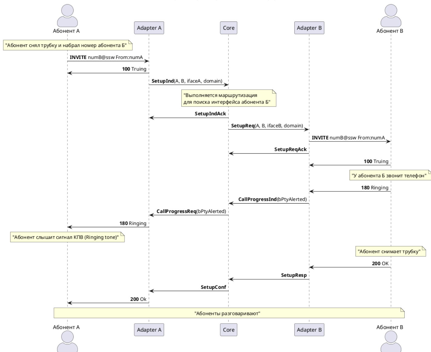
Базовый вызов по протоколу SIP в режиме "enblock", упрощенный вид
