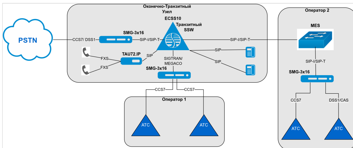
Рисунок 7 — Пример построения оконечно-транзитного узла связи на основе ECSS-10
