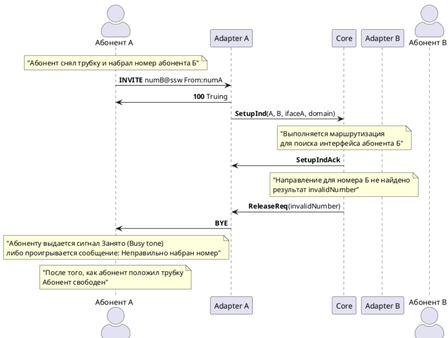
Рисунок 17 — Неуспешный вызов по причине того, что номер Б не существует
