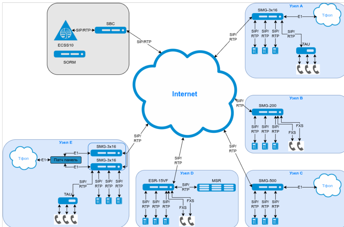
Рисунок 1 – Типовая схема организации распределенной отказоустойчивой сети
