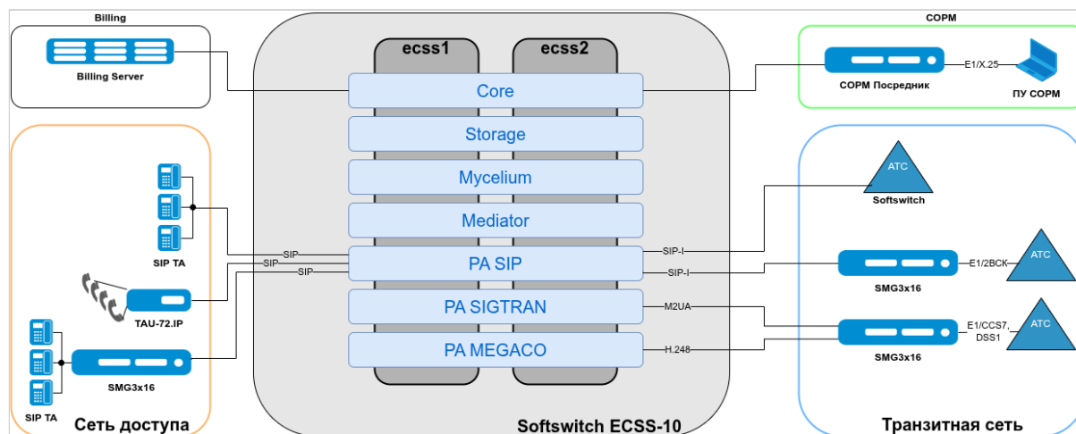
Рисунок 1 – Функциональный состав ПО системы ECSS-10
