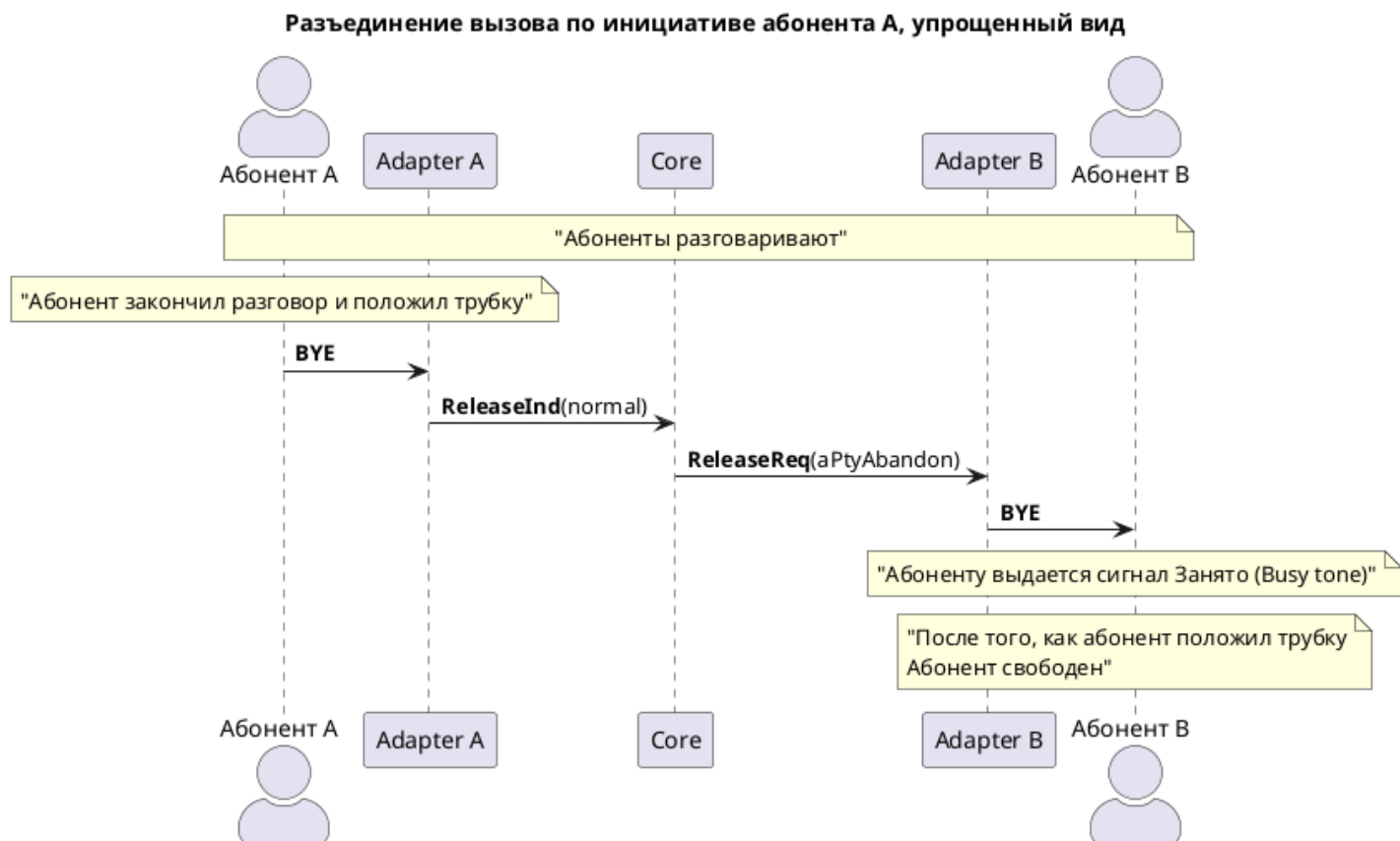
Рисунок 14 — Разъединение вызова по инициативе абонента А, упрощенный вид
