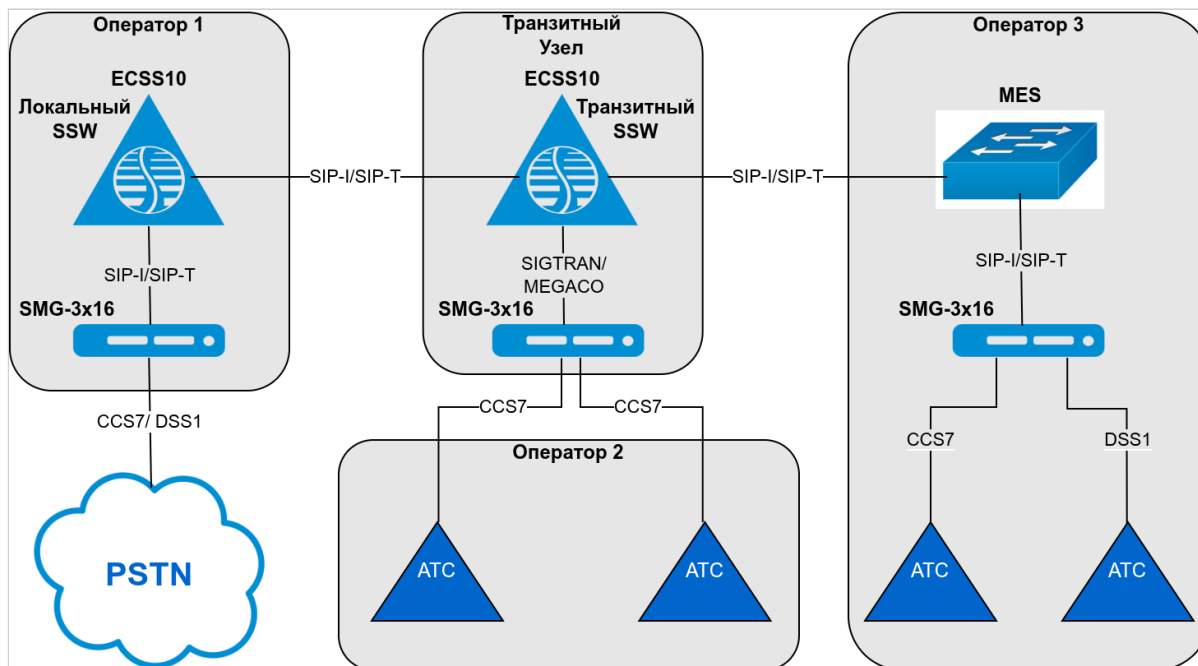
Рисунок 6 — Пример построения зонального узла связи на основе ECSS-10
