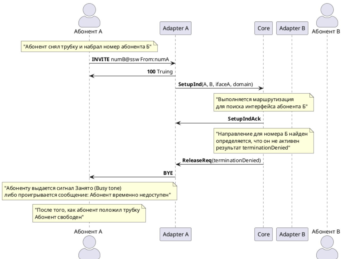
Рисунок 18 – Неуспешный вызов по причине того, что интерфейс абонента Б не активен
