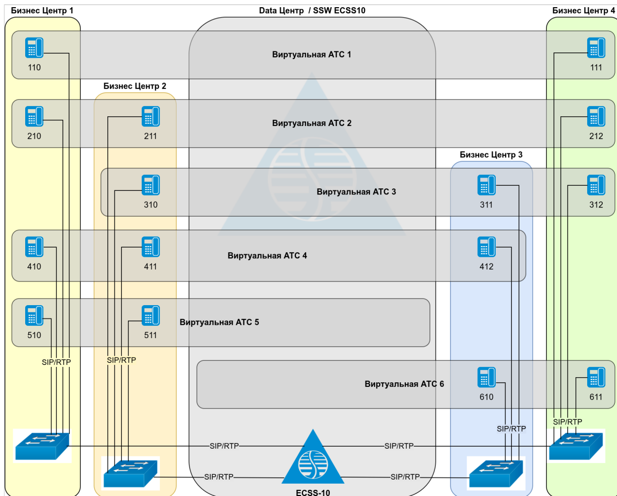
Рисунок 8 – Пример построения SaaS платформы на основе ECSS-10
