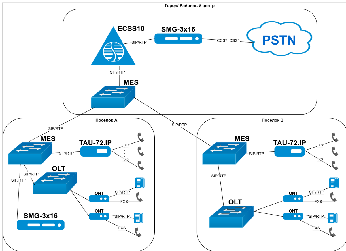
Рисунок 5 – Пример построения сельского узла связи на основе ECSS-10
