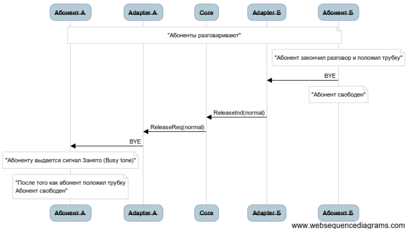
Рисунок 17 – Разъединение вызова по инициативе абонента Б, упрощенный вид
