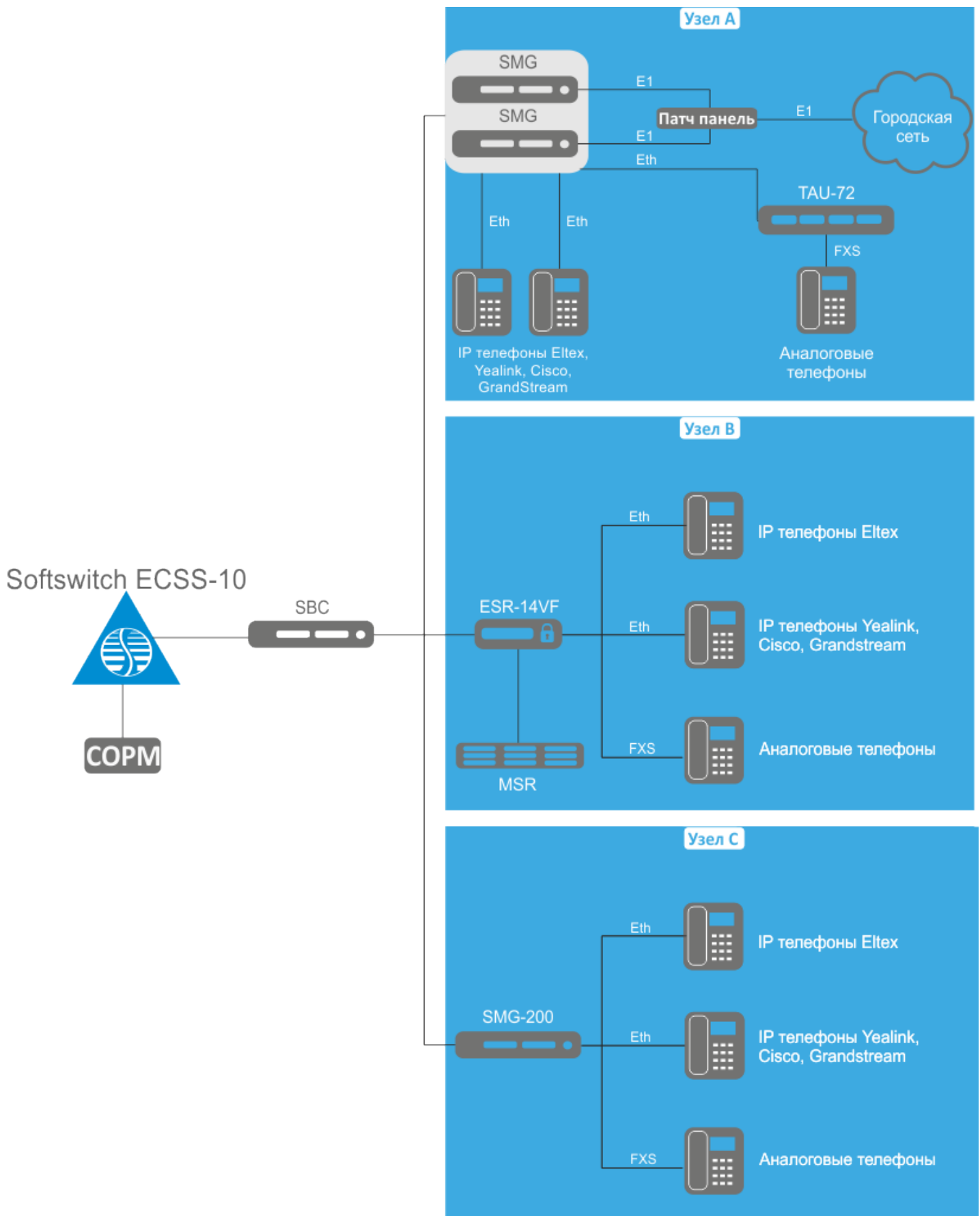
Рисунок 33 – Типовая схема организации распределенной отказоустойчивой сети
