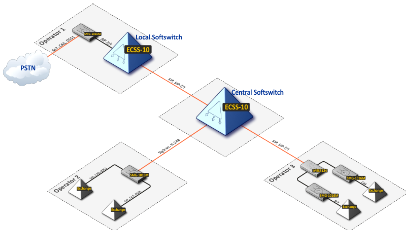
Рисунок 8 – Пример построения зонового узла связи на основе ECSS-10
