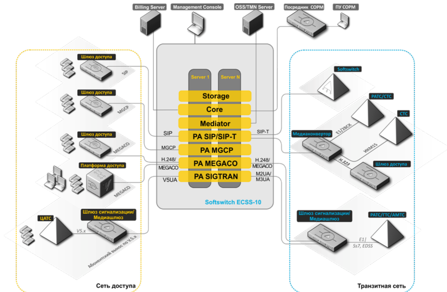
Рисунок 14 – Функциональный состав ПО системы ECSS-10
