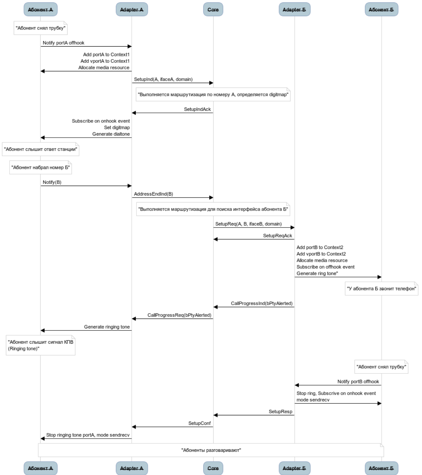
Рисунок 18 – Базовый вызов по протоколу H.248/Megaco в режиме "enblock", упрощенный вид
