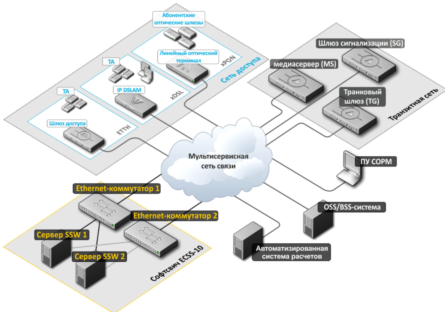
Рисунок 1 – Пример схемы включения комплекса ECSS-10
