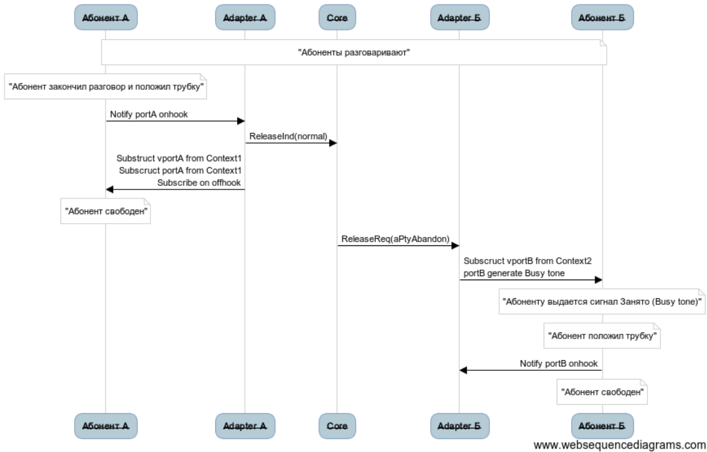
Рисунок 19 – Разъединение вызова по инициативе абонента А по протоколу H.248/Мегасо, упрощенный вид
