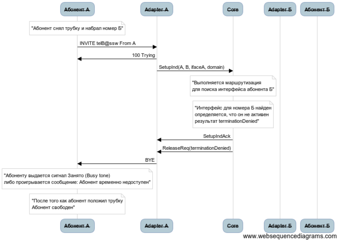
Рисунок 23 – Неуспешный вызов по причине того, что интерфейс абонента Б не активен
