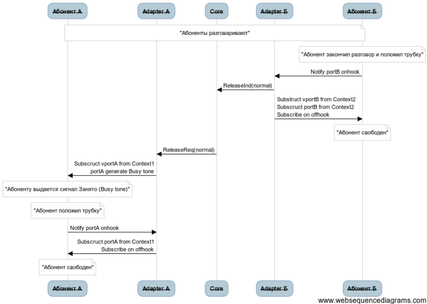
Рисунок 20 – Разъединение вызова по инициативе абонента Б по протоколу H.248/Megaco, упрощенный вид
