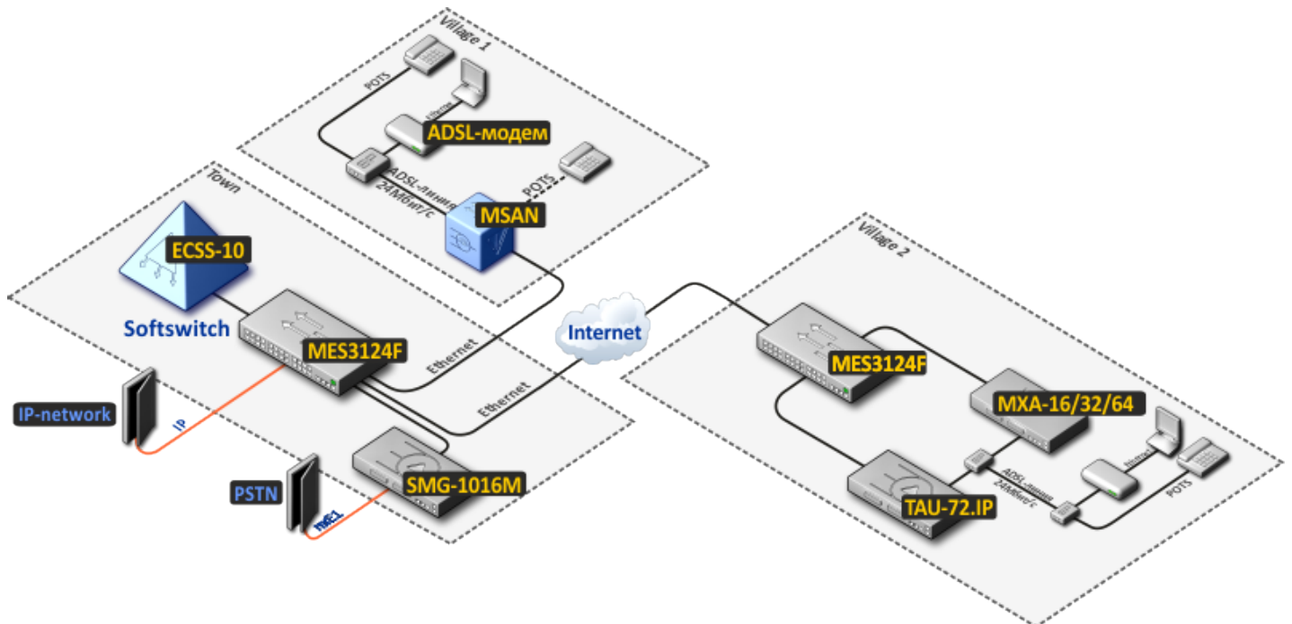
Рисунок 7 – Пример построения сельского узла связи на основе ECSS-10
