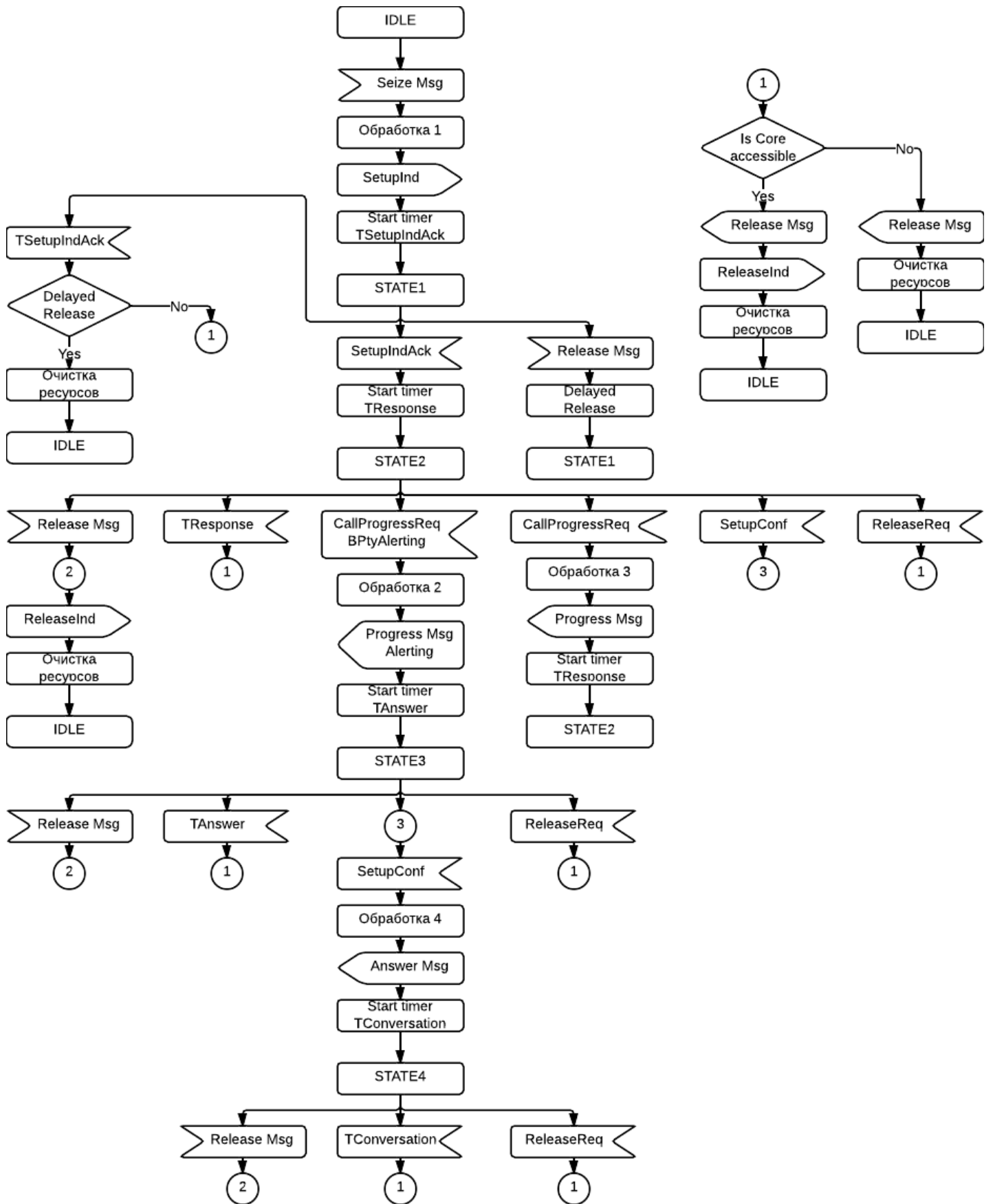
Рисунок 24 – Диаграмма работы originating кластера Adapter (Adapter A)
