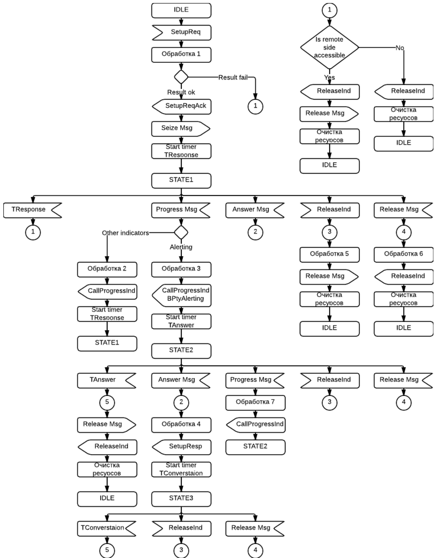
Рисунок 26 – Диаграмма работы terminating кластера Adapter (Adapter Б)
