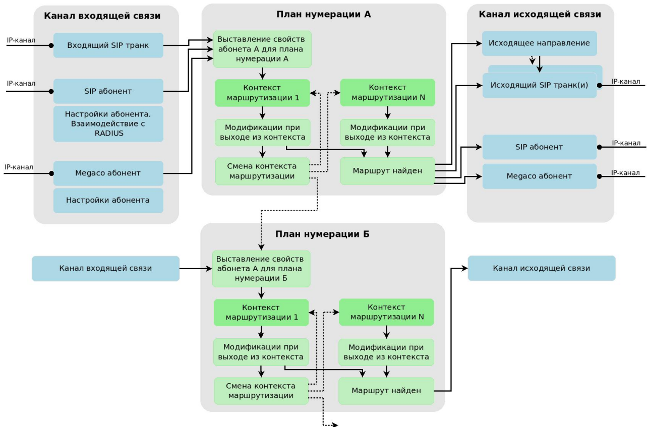
Рисунок 1 — Общая схема прохождения телефонного вызова
