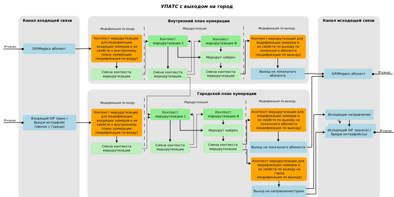
Рисунок 2 – Общая схема построения контекстов маршрутизации
