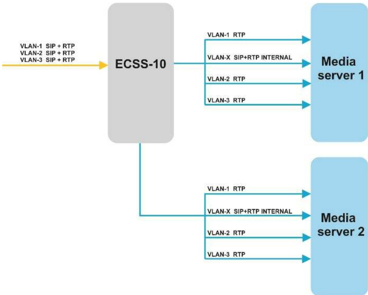
Рисунок 2 — Типовой случай распределенного медиасервера
