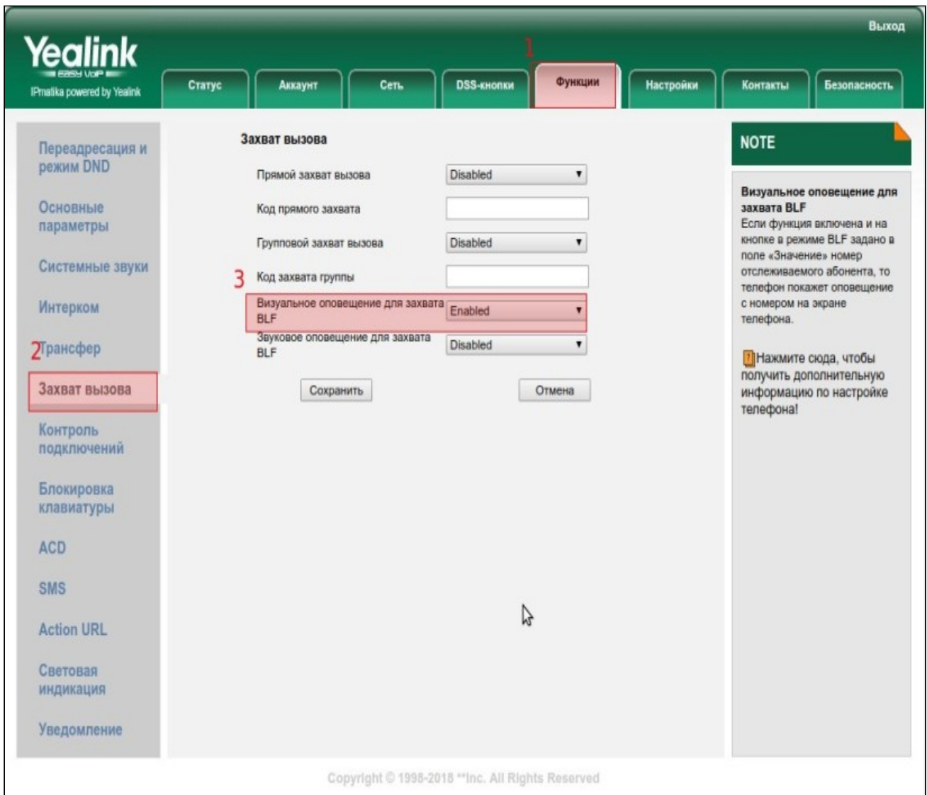
Рисунок 9. Настройка визуального оповещения для захвата BLF
