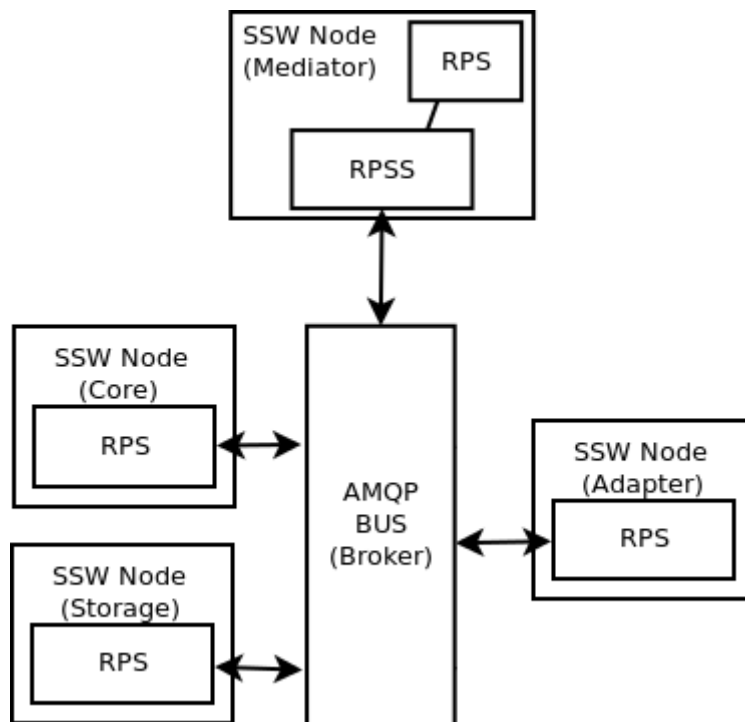
Рисунок 1 — Общая схема взаимодействия кластера Mediator с другими кластерами системы В качестве источников статистики могут выступать следующие компоненты ECSS-10:
