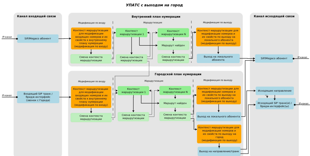
Рисунок 2 – Общая схема построения контекстов маршрутизации
