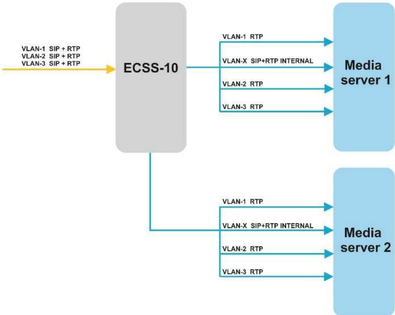
Рисунок 2 — Типовой случай распределенного медиасервера
